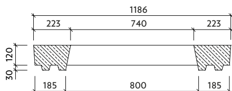
Ukázka tvaru
