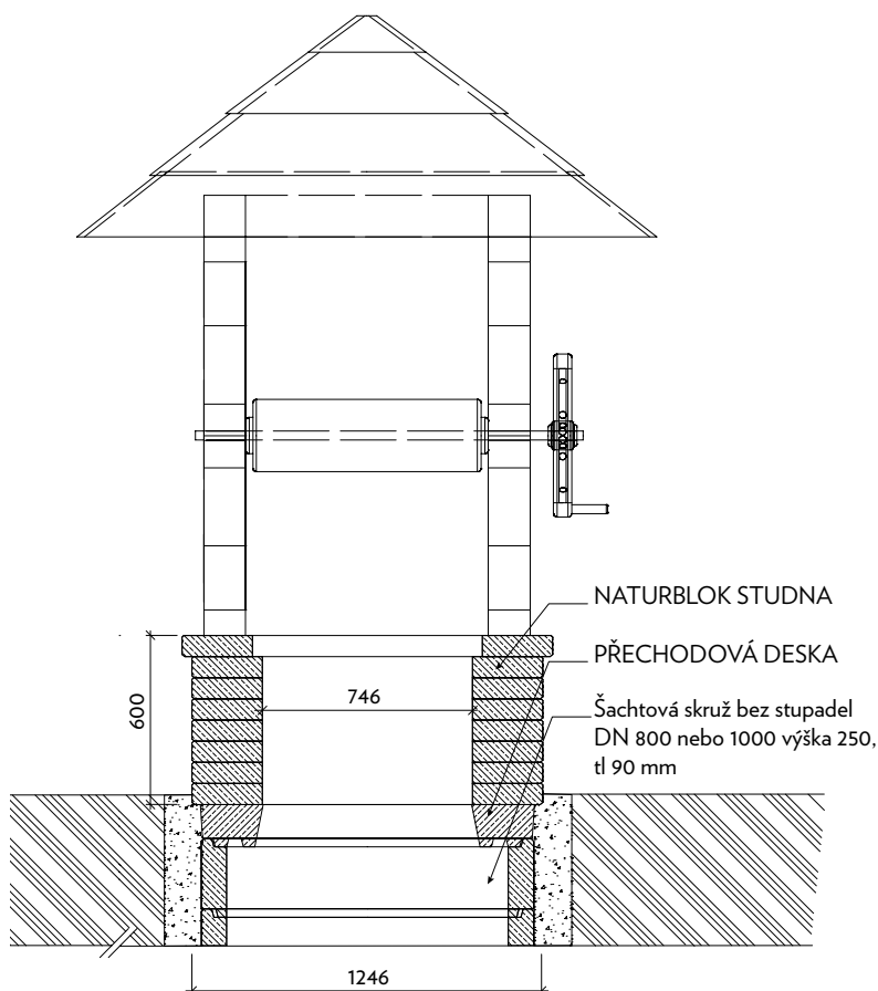
Ukázkový řez
