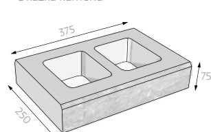
kámen C 75 mm
