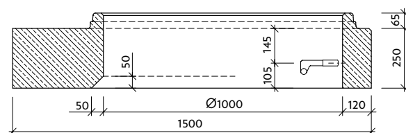
Řez atypickou roznášecí deskou - OPRAVY PRAHA
