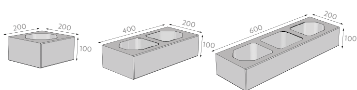
skladba 3 kamenů
