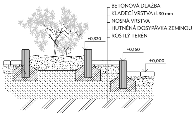
Řez a-a':
