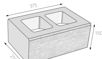
kámen C 150 mm
