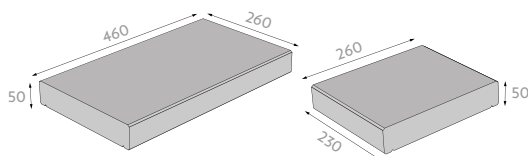
stříška - základní kámen SOLOBLOK/NEWBLOK
