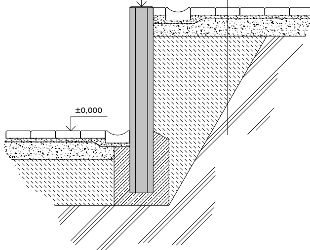
Řez a-a': +1,000 ±0,000 BETONOVÁ DLAŽBA KLADEČÍ VRSTVA tl. 30 mm NOSNÁ VRSTVA HUTNĚNÁ DOSYPÁVKA ZEMINOU ROSTLÝ TERÉN
