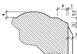
Řez hranou (v 80 mm)
