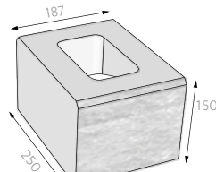
kámen A 150 mm
