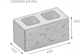
jednostranně štípaný
