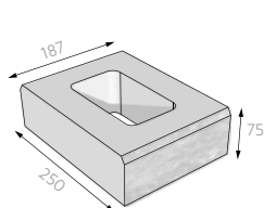
kámen A 75 mm
