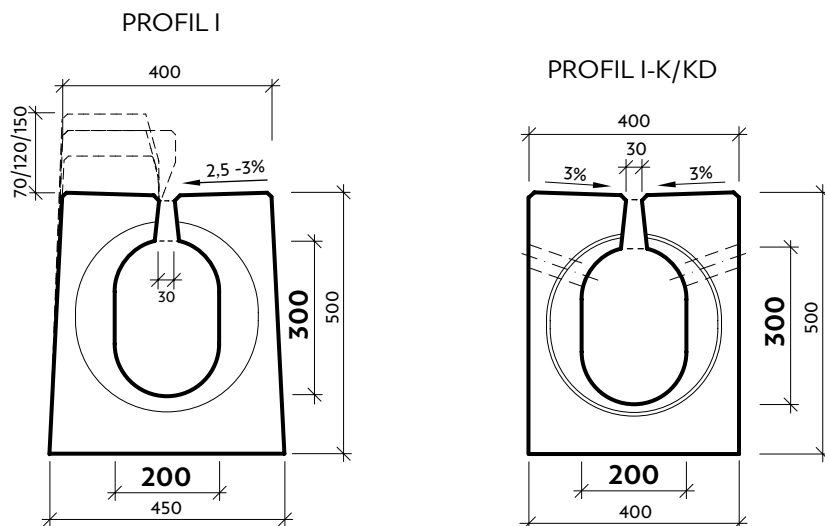
Ukázka základních prvků
