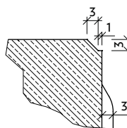
Řez hranou
