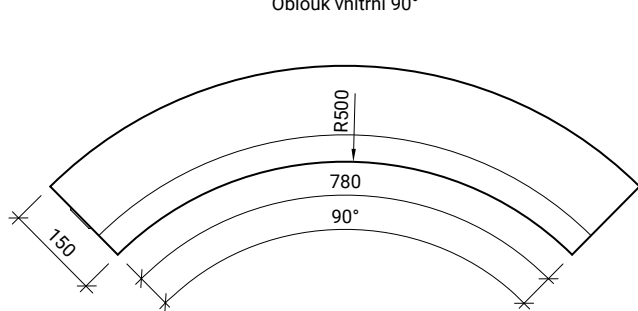
Obrubník silniční H 25 R 0,5
