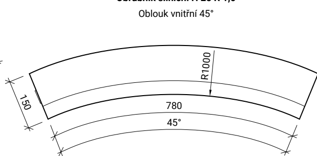
Obrubník silniční H 25 R 1,0
